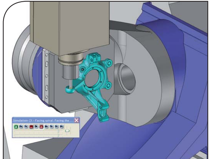
Simulation intégrée de l'ensemble des équipements (outils, outillage, machine) pendant le processus de programmation.
