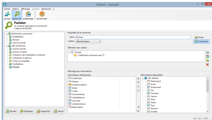
Vue de l'écran d'élaboration des recherches
