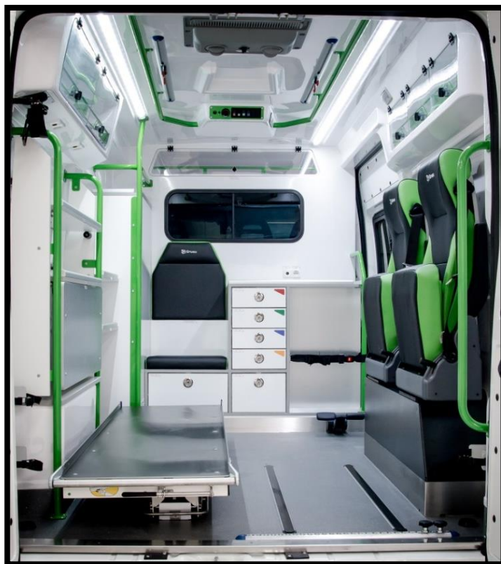
Vue cellule, rails TPMR en option
