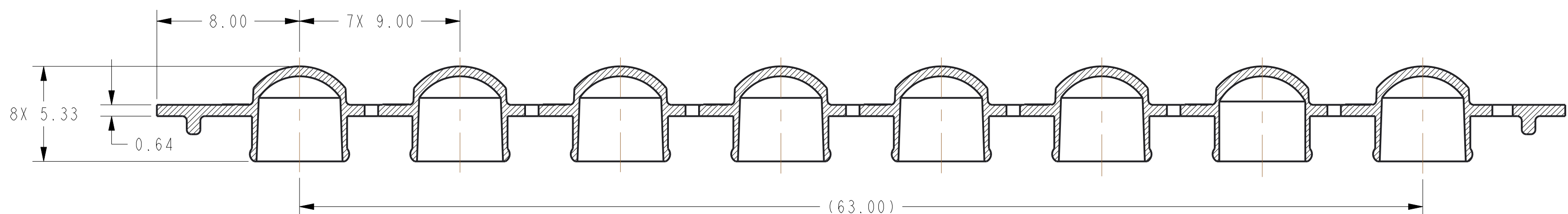
SECTION A-A
