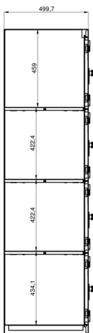
COUPE A-A
