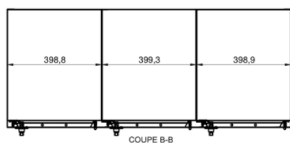
COUPE B-B
