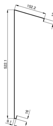
COUPE B-B
