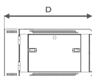
Vue gauche
