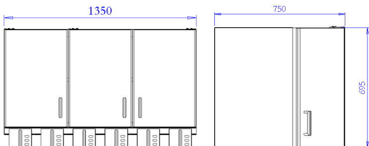
MMU3P + MMUB2
