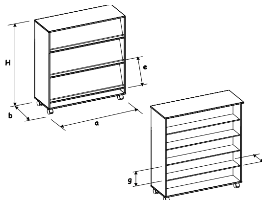
Roulettes double galets
