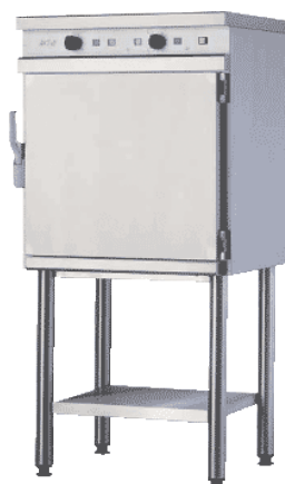
FOUR DE REMISE EN TEMPERATURE CFE 707 RT
