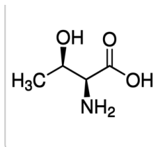
T4071 L-Threonine
