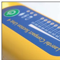
Caractéristiques de l'écran de contrôle: Bouton marche/arrêt, indicateur d'alimentation externe, indicateur batterie faible, réglage niveau de vide visible par LED
