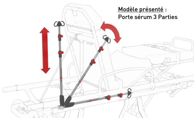
Porte sérum repliable 2 ou 3 parties
