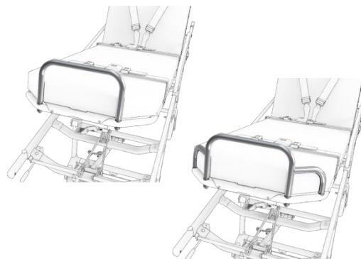
Barrière de pieds S10.001 (Standard) S10.016 (Renforcée)
