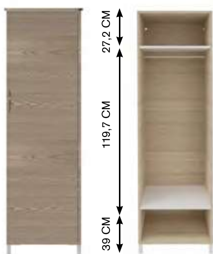
Armoire 1 porte 74-0554M 60x56x190 cm 80,5 kg
