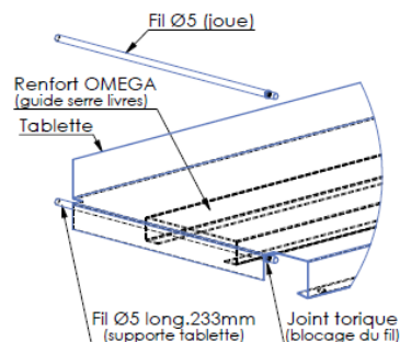
DÉTAIL D
