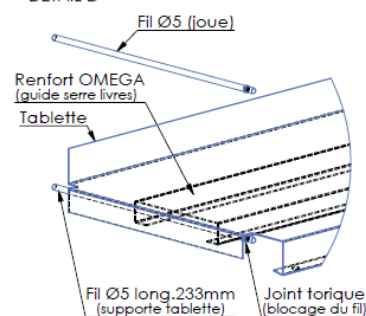
DÉTAIL D
