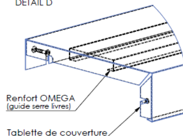
DÉTAIL D
