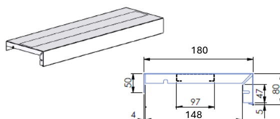
DÉTAIL D
