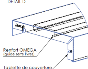
DÉTAIL D
