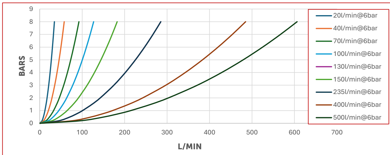
Courbe débit / pression pour les Multiflow (à sélection de débit)
