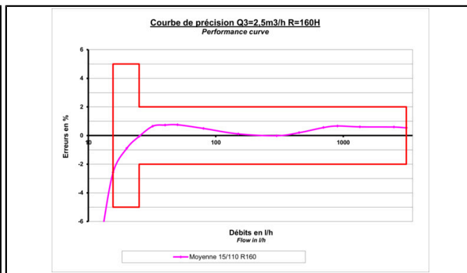
DN15 - composite
